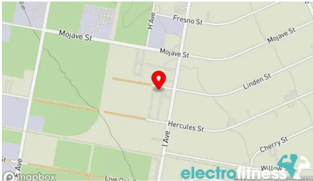
Epicentre map
